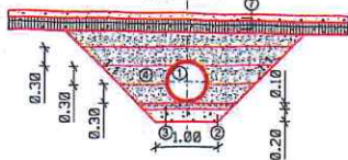
ĒZ D-D'
