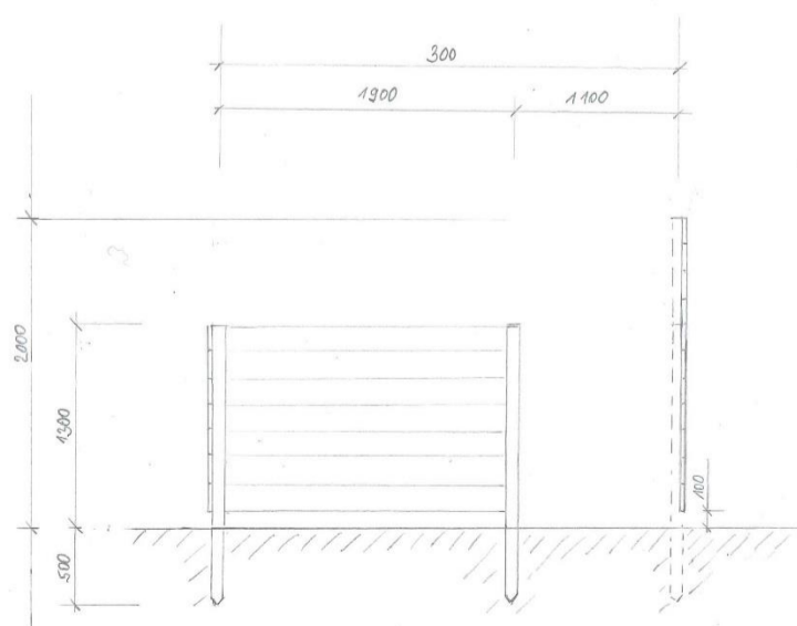
ŘEZ A-A'
